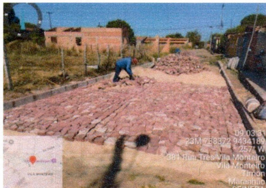
5.3 PAVIMENTAÇÃO EM PARALELEPÍPEDO
