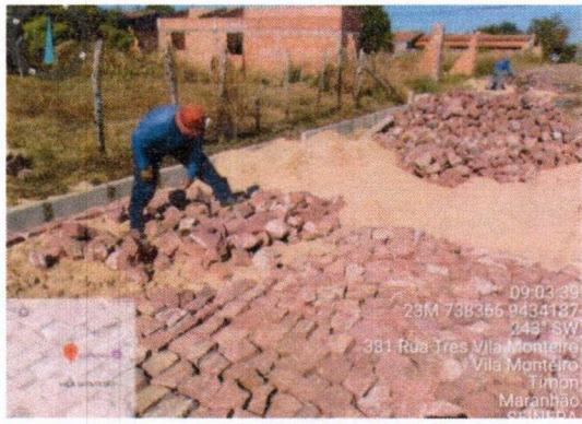
5.3 PAVIMENTAÇÃO EM PARALELEPÍPEDO
