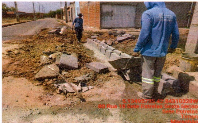
8.1 Assentamento de guia
