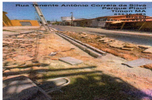
8.1 Assentamento de guia
