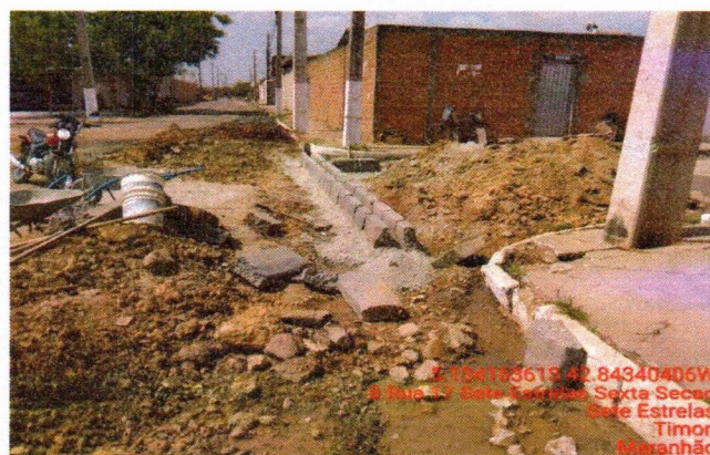
8.1 Assentamento de guia
